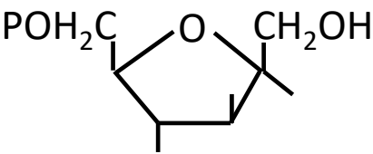
fructose-6-P
